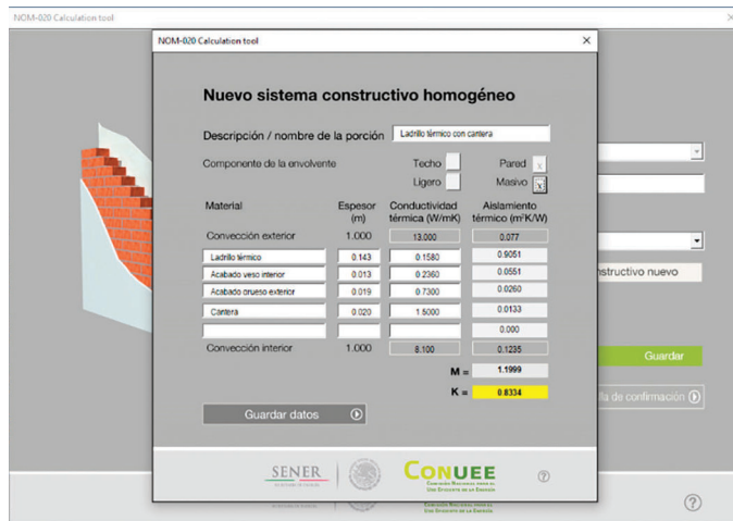
Figura 5. Captura de los sistemas constructivos para muros de la vivienda A
