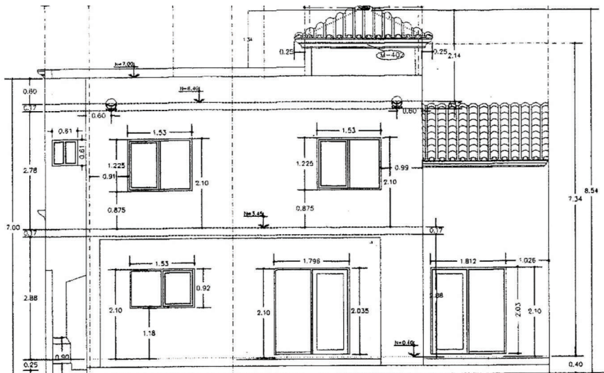
Figura 3. Fachada principal de prototipo B
