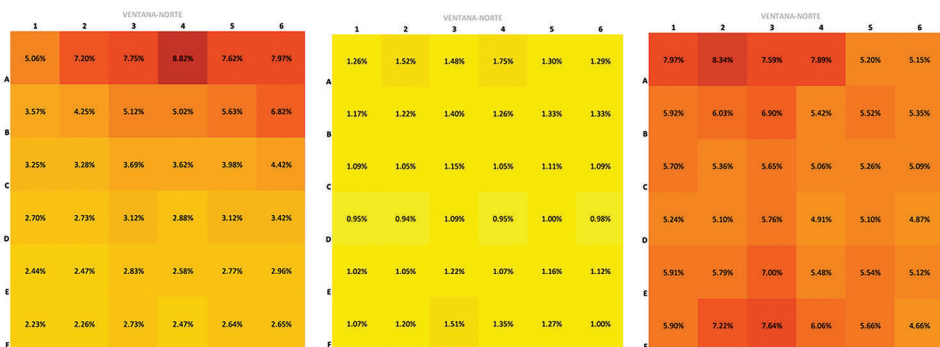
Figura 9. Planta del aula tipo en el modelo a escala y distribución de factor de iluminación natural, un día de verano a las 8, 13 y 17 hr
