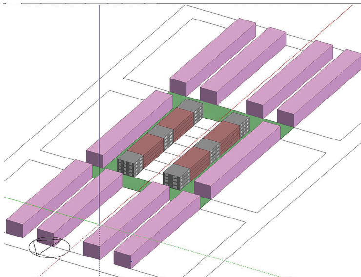
Figura 21. Ejemplo de modelado de bloques de edificios y contexto para escenario densificado B2 de la muestra de morfología urbana (MMU) de la colonia Modelo
