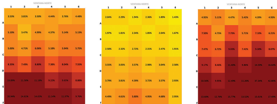
Figura 8. Planta del aula tipo en el modelo a escala y distribución de factor de iluminación natural, un día de invierno a las 8, 13 y 17 hr
