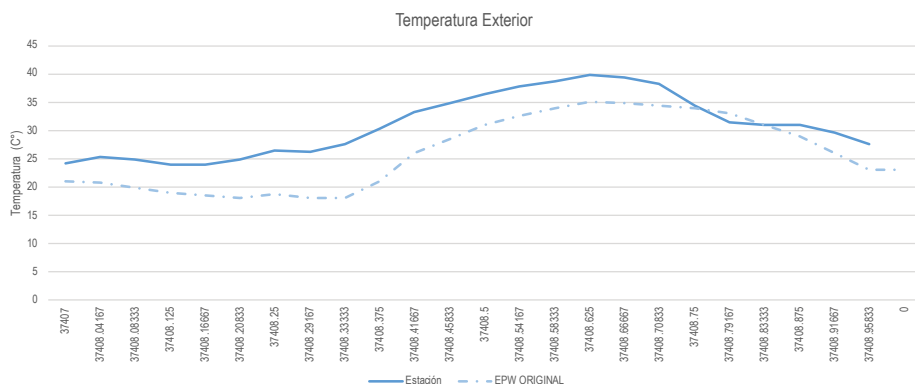
Figura 18. Temperatura Exterior BS. Comparación entre archivo climático EPW y monitoreo en tiempo real para el 1 de mayo del 2021
