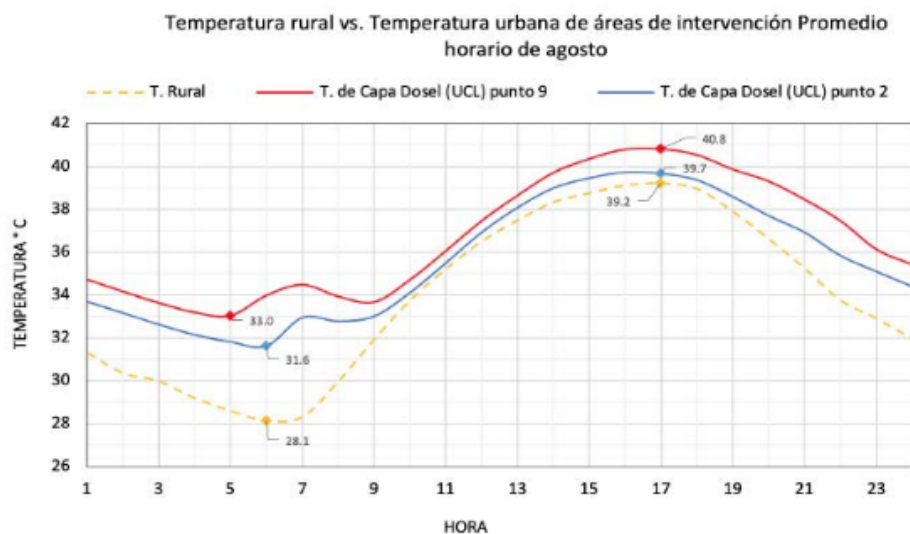
GRÁFICA V.3. Perfil de temperatura rural y urbana de verano
