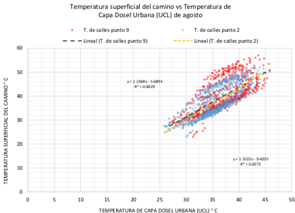
GRÁFICA V.7. Dispersión de temperatura superficial del camino y temperatura de UCL
