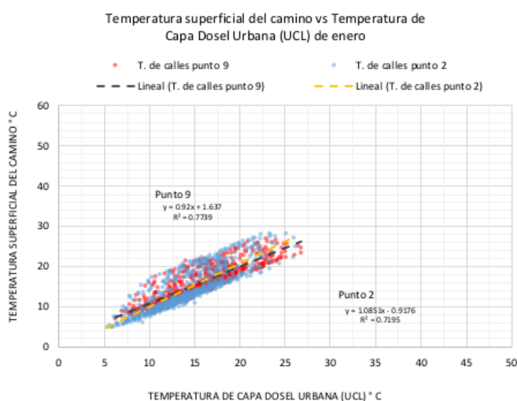
GRÁFICA V.12. Dispersión de temperatura superficial del camino y temperatura de UCL
