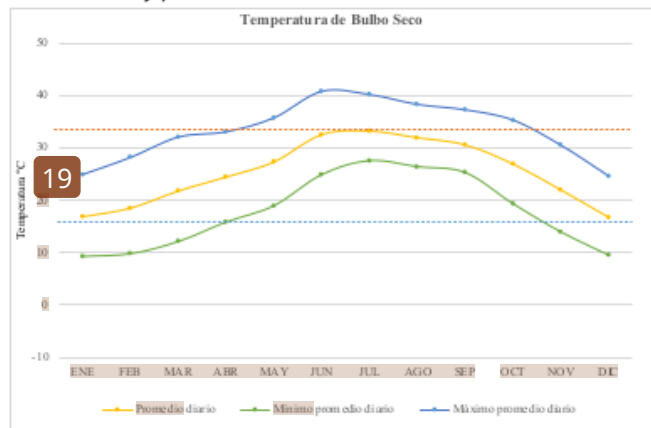
GRÁFICA IV.1. Temperatura de bulbo seco en promedio diario, promedio mínimo y promedio máximo de Hermosillo, Sonora
