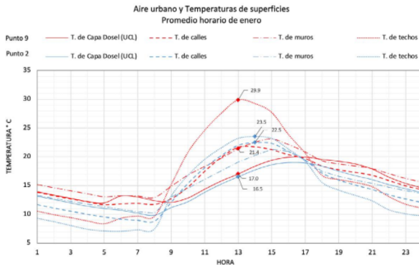
GRÁFICA V.10. Aire urbano y temperaturas de superficies de invierno
