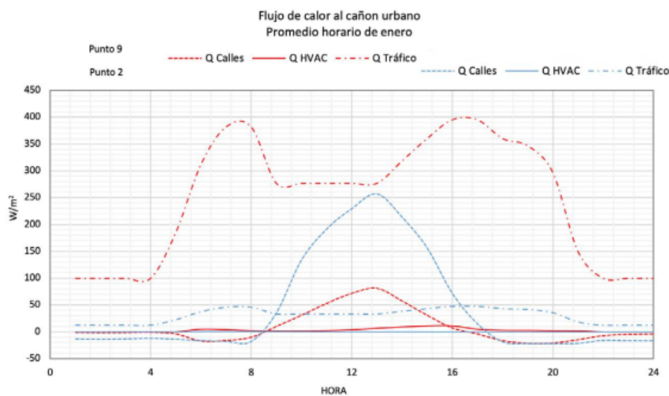
GRÁFICA V.11. Flujo de calor al cañón urbano de calles, HVAC y tránsito vehicular
