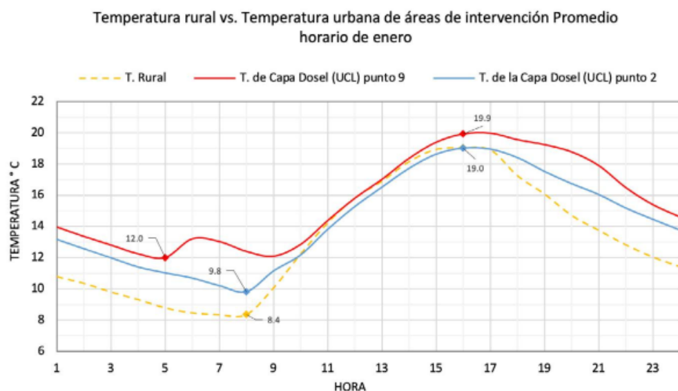
GRÁFICA V.8. Perfil de temperatura rural y urbana de invierno
