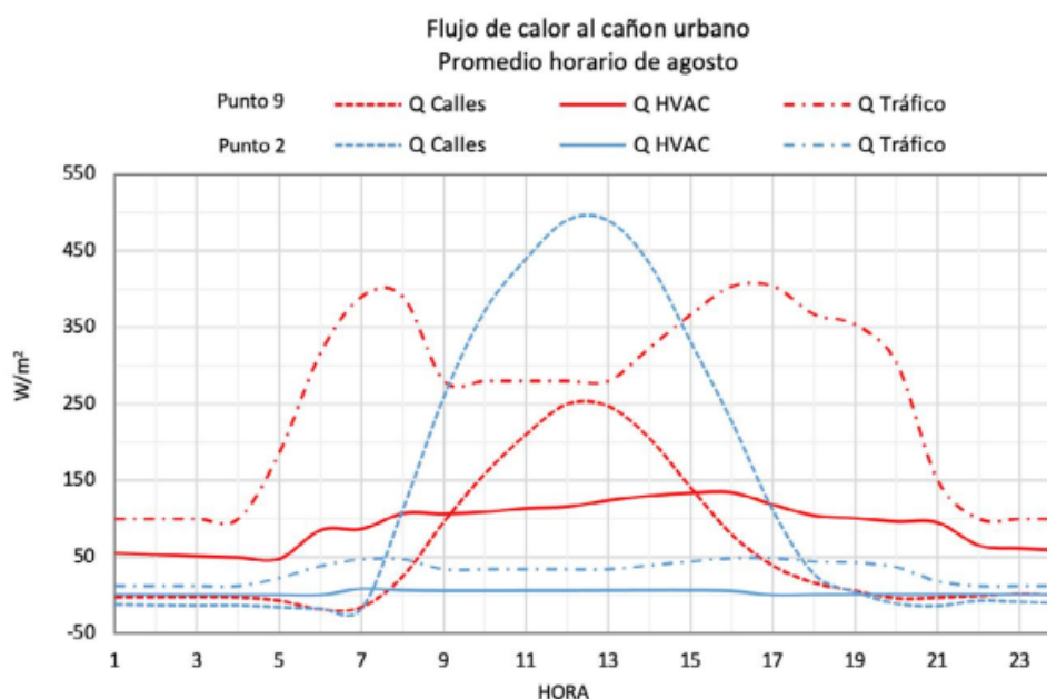
GRÁFICA V.6. Flujo de calor al cañón urbano de calles, HVAC y tránsito vehicular
