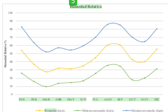
GRÁFICA IV.2. Humedad relativa en promedio diario, promedio mínimo y promedio máximo de Hermosillo, Sonora.
