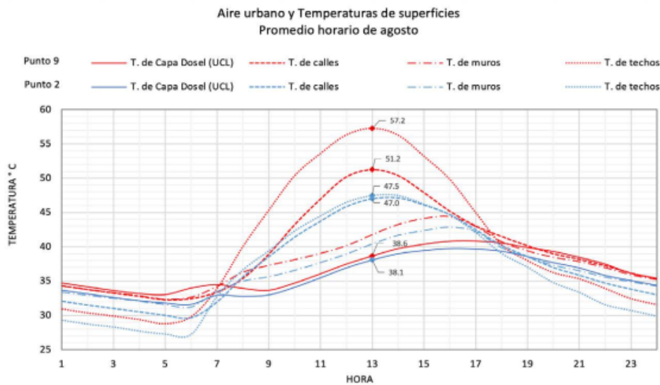
GRÁFICA V.5. Aire urbano y temperaturas de superficies de verano
