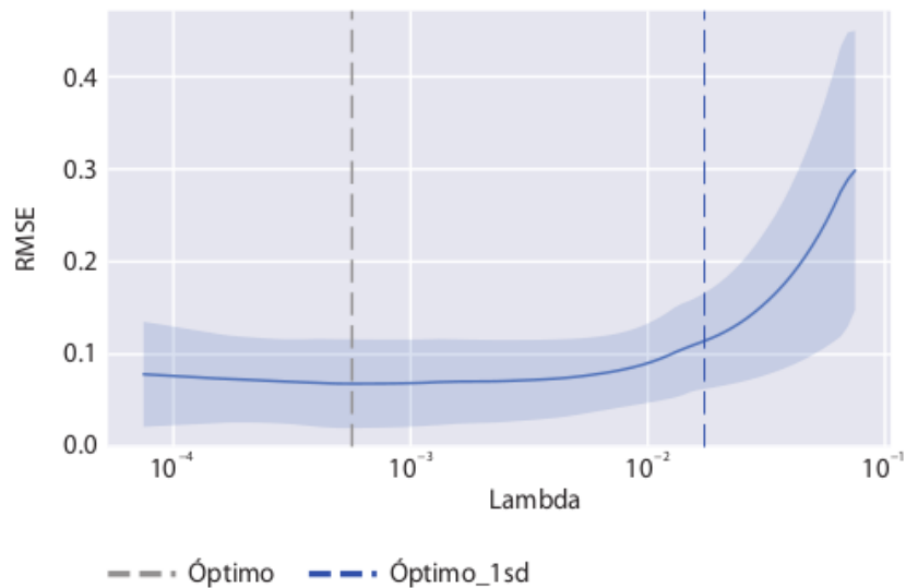
Gráfica 13.5. Evolución del error con validación cruzada (CV) en función de la regularización
