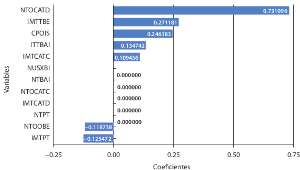
Gráfica 13.8. Coeficientes de las variables explicativas por el método LASSO
