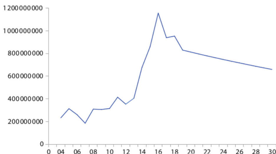
Gráfica 8.6. Pronóstico contribuciones 2020-2030
