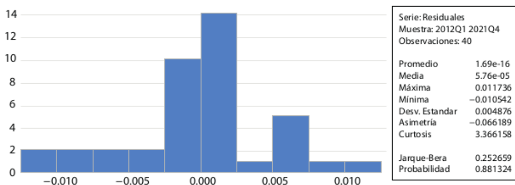
Gráfica 7.1. Histograma de los residuos y prueba de normalidad Jarque-Bera
