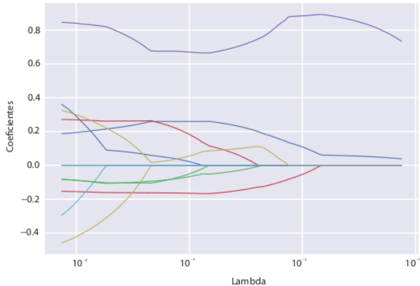
Gráfica 13.4. Coeficientes del modelo en función de la regularización
