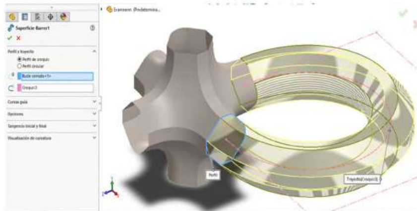
Figura 9.16. Realizar barrido por superficie
