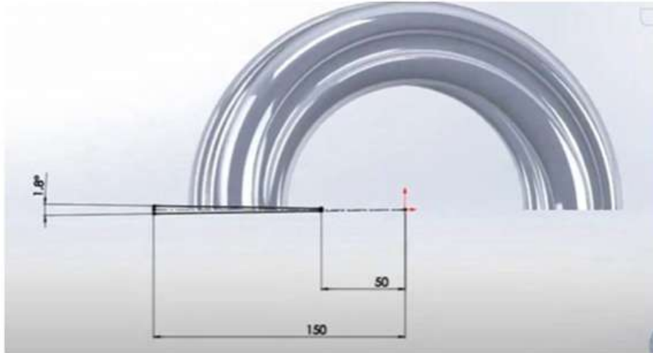
Figura 3.46. Realizar un croquis para corte
