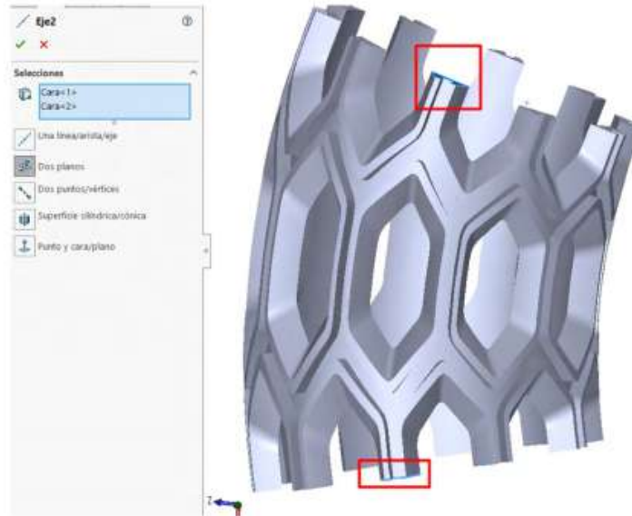
Figura 4.72. Realizar render con aplicación de materiales
