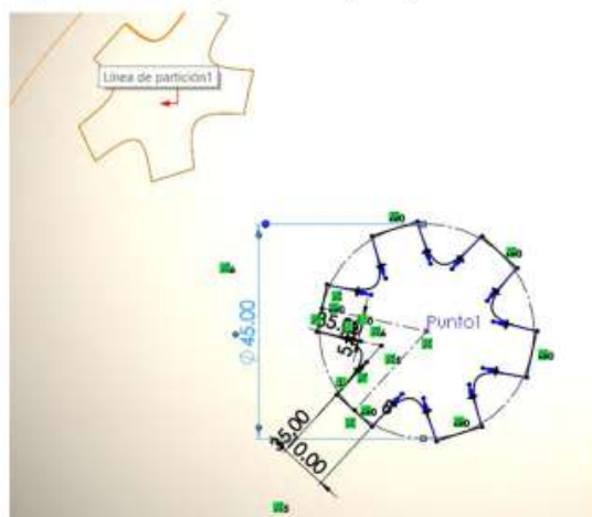
Figura 10.13. Proyectar croquis a plano inclinado
