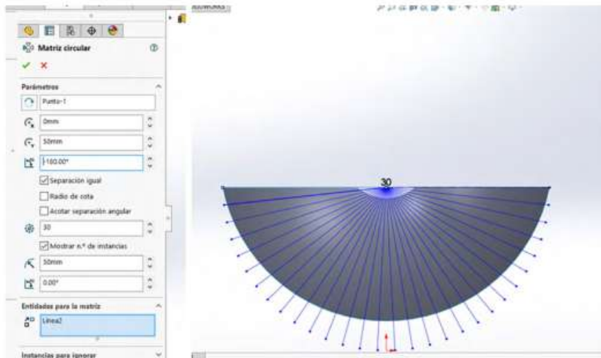
Figura 5.14. Patrones de la matriz
