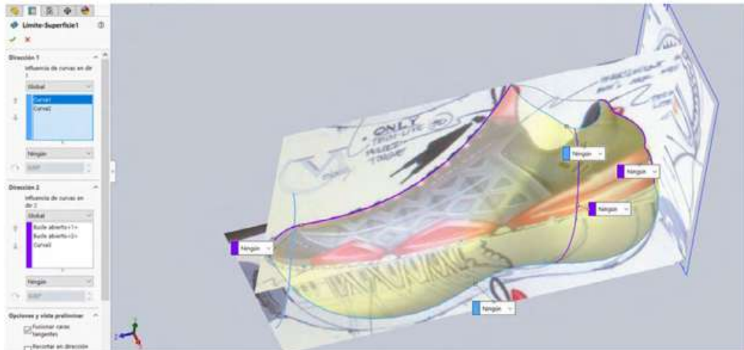
Figura 8.16. Realizar operación limite por superficie, mediante curvas guías
