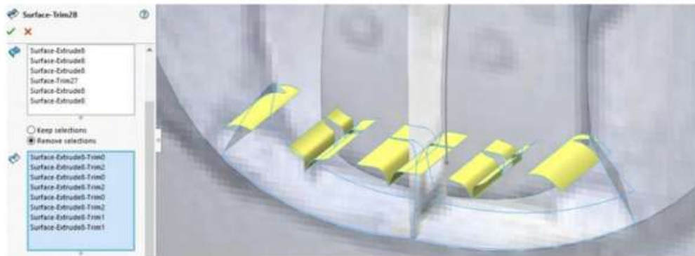
Figura 11.116. Recortar por superficie las caras externas
