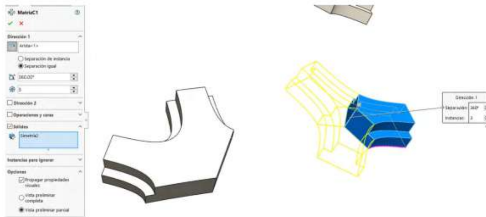
Figura 10.31. Realizar matriz circular
