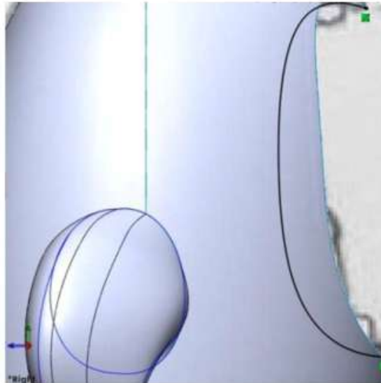
Figura 11.95. Realizar croquis libre para cerrar operación
