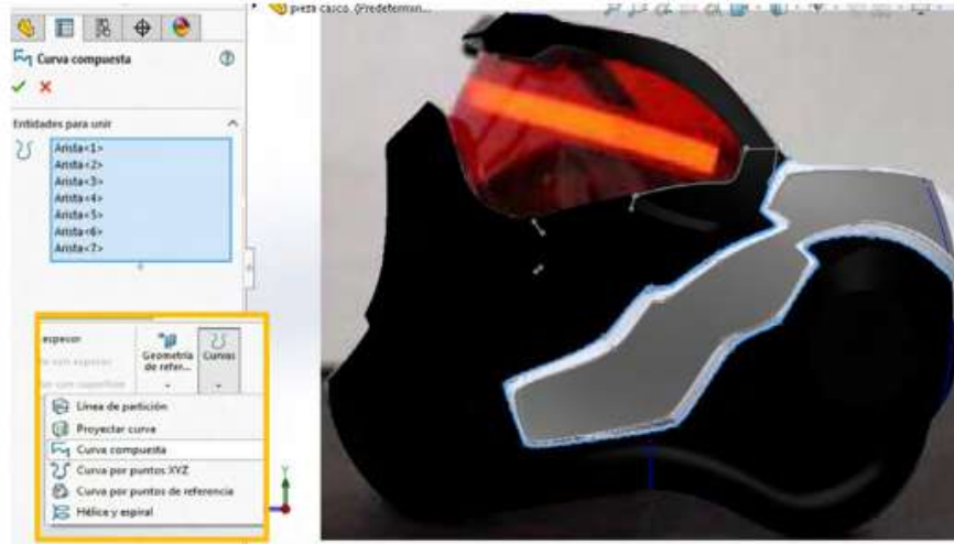
Figura 1.81. Mediante la opción de curva compuesta
