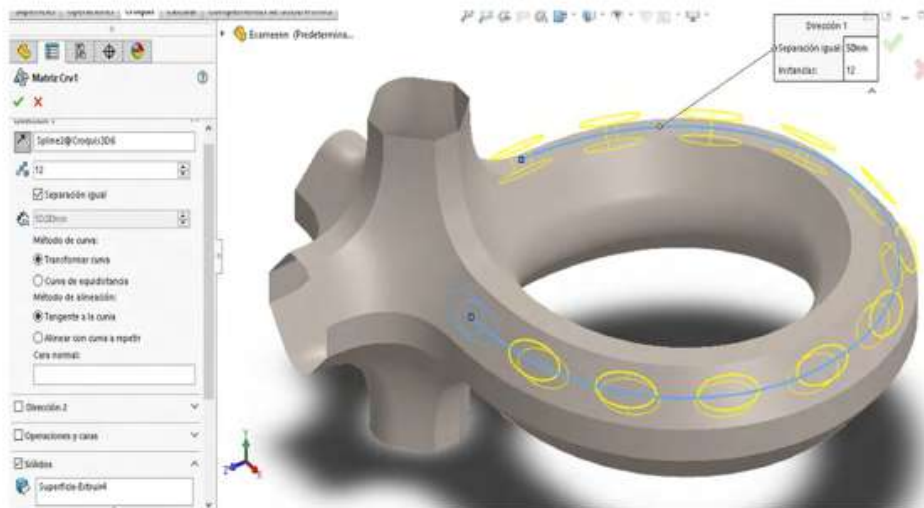
Figura 9.20. Realizar matriz por curva conducida
