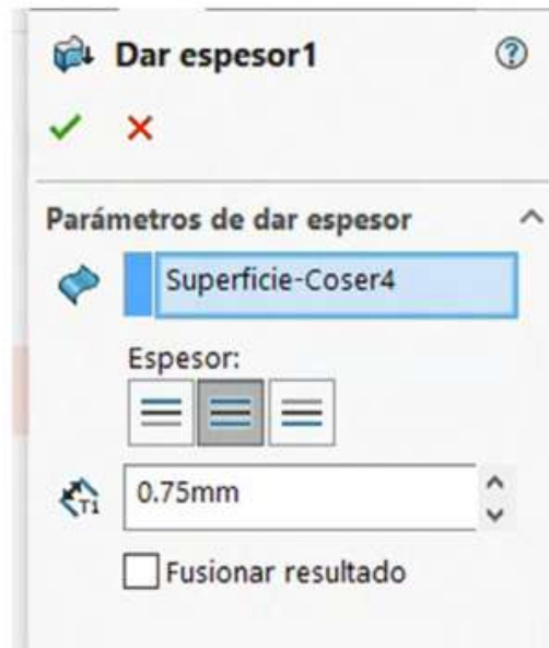
Figura 5.30. Realizar operación de espesor
