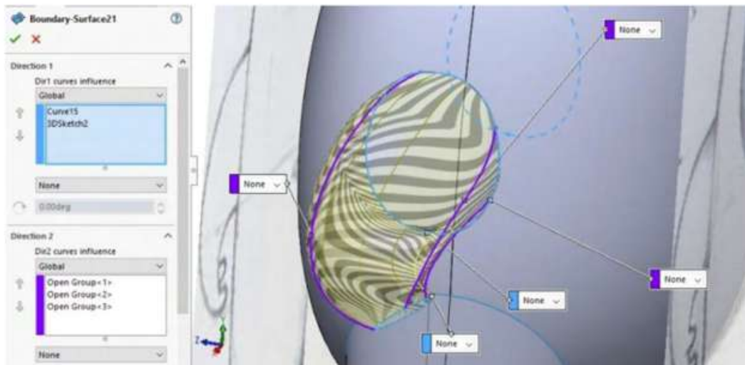
Figura 11.84. Realizar operación de relleno por superficies de limitante
