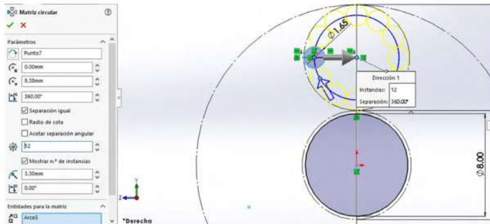
Figura 2.4. Matriz para cuerpo múltiple
