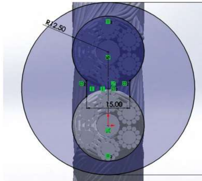
Figura 2.12. Dimensiones y relaciones inteligentes en vertical
