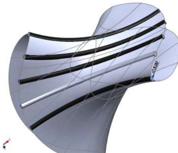
Figura 11.17. Realizar croquis para barrer por superficie
