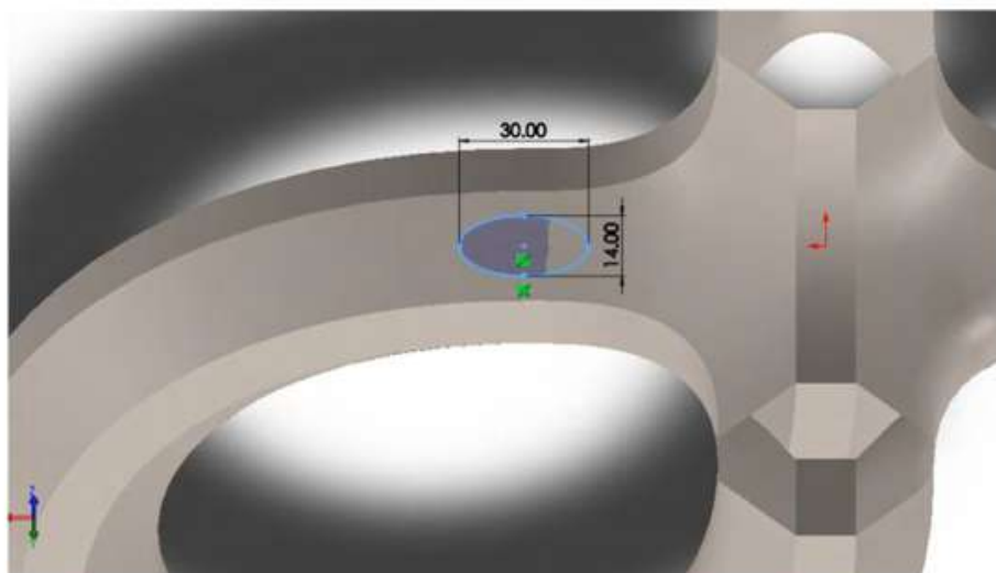
Figura 9.17. Realizar croquis para corte
