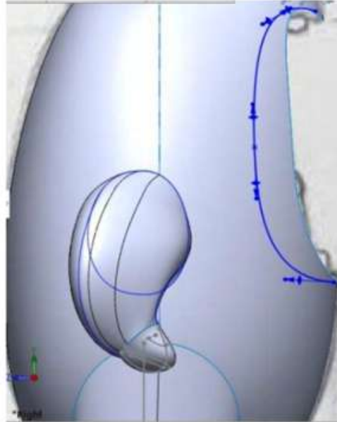
Figura 11.93. Realizar croquis libre para dar profundidad a boca
