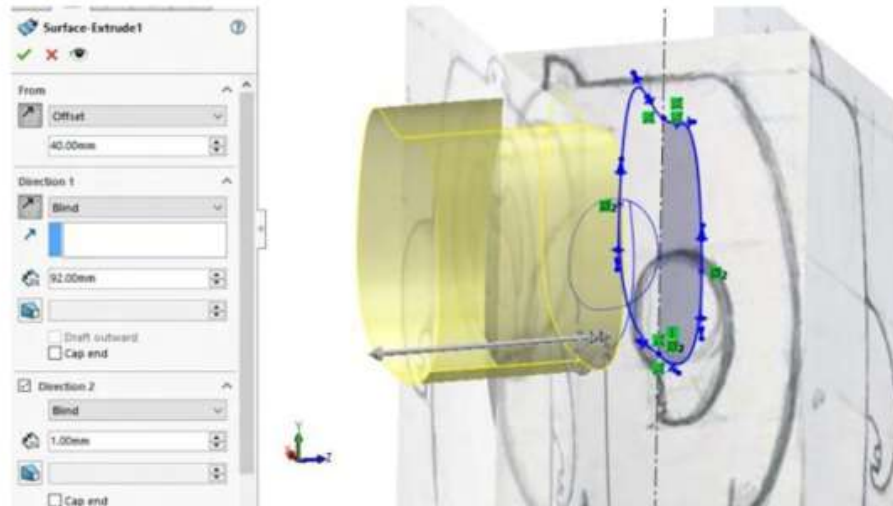
Figura 11.91. Realizar operación de extruir por superficie
