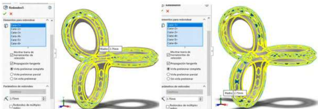
Figura 9.25. Aplicar redondeos en aristas
