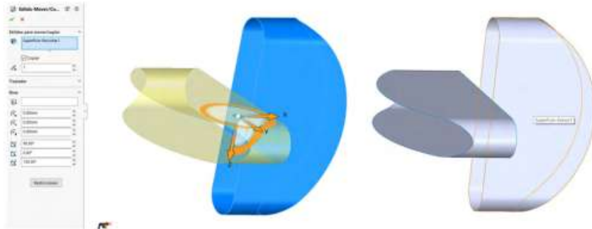
Figura 11.6. Mediante operación mover/copiar
