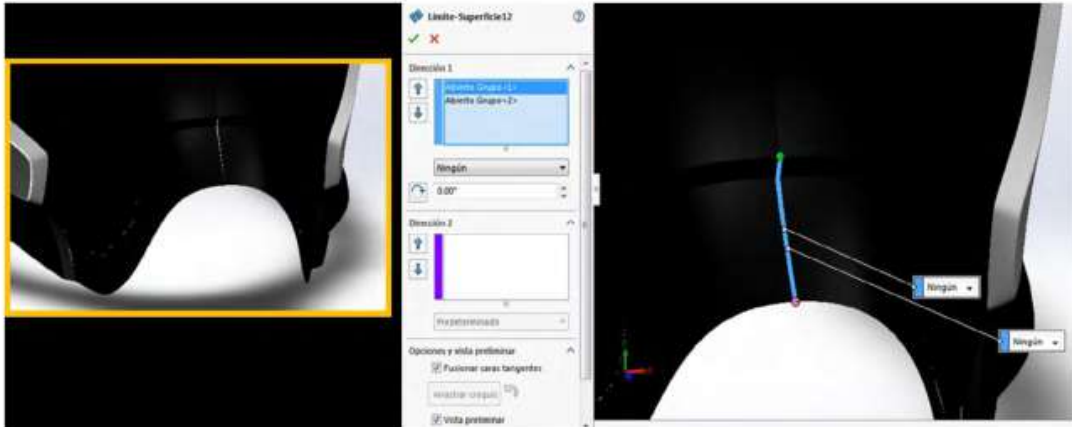
Figura 1.137. Mediante la opción de superficie limitante
