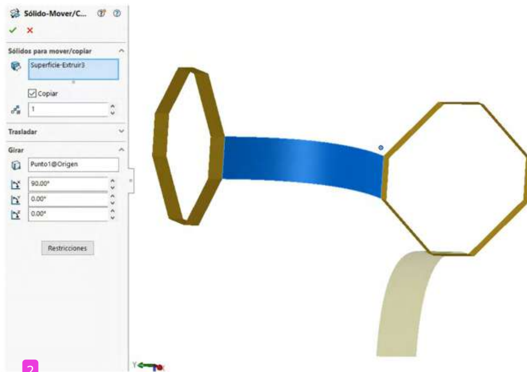
Figura 9.7. Realizar operación mover/copiar opción por ángulo
