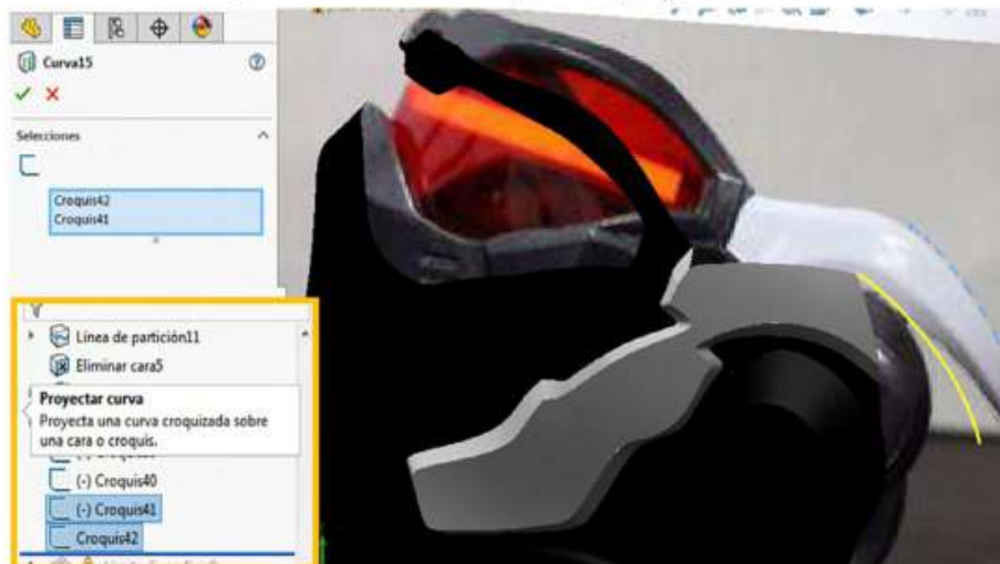
Figura 1.98. Mediante la opción de proyectar curva
