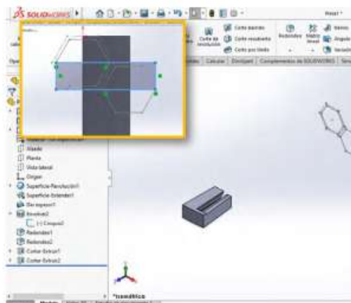
Figura 3.7. Insertar rectángulo por cada vértice del polígono
