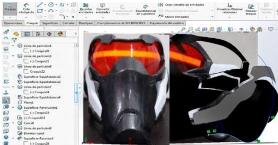
Figura 1.63. Por vista lateral mediante spline
