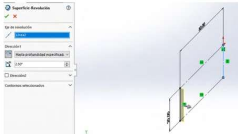
Figura 3.3. Dimensionando y revolución
