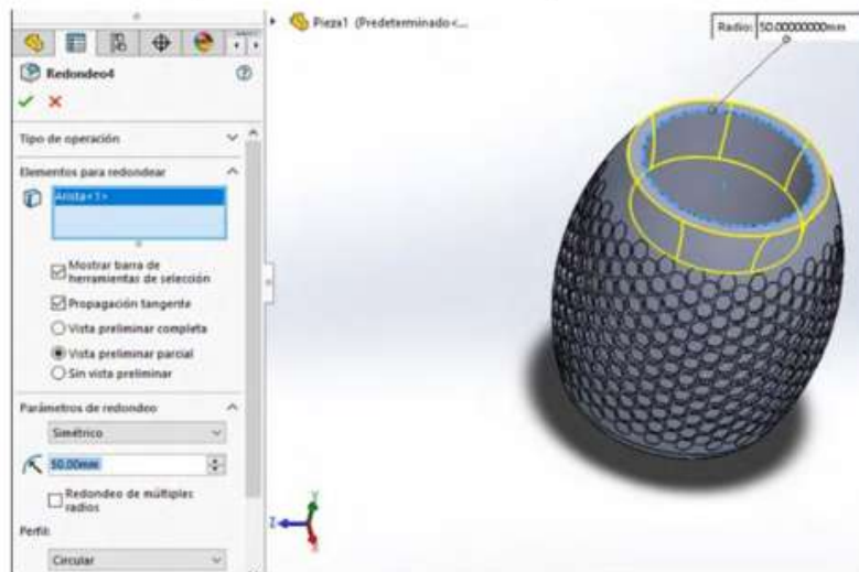
Figura 3.23. Realizar redondeos parte inferior
