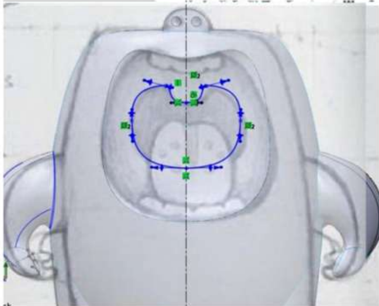
Figura 11.97. Realizar croquis libre por spline para imitar garganta según modelo
