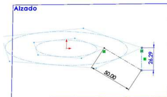
Figura 10.3. Realizar líneas auxiliares
