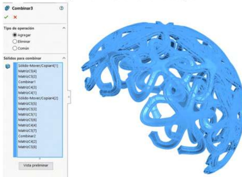
Figura 10.47. Realizar combinar cuerpos
