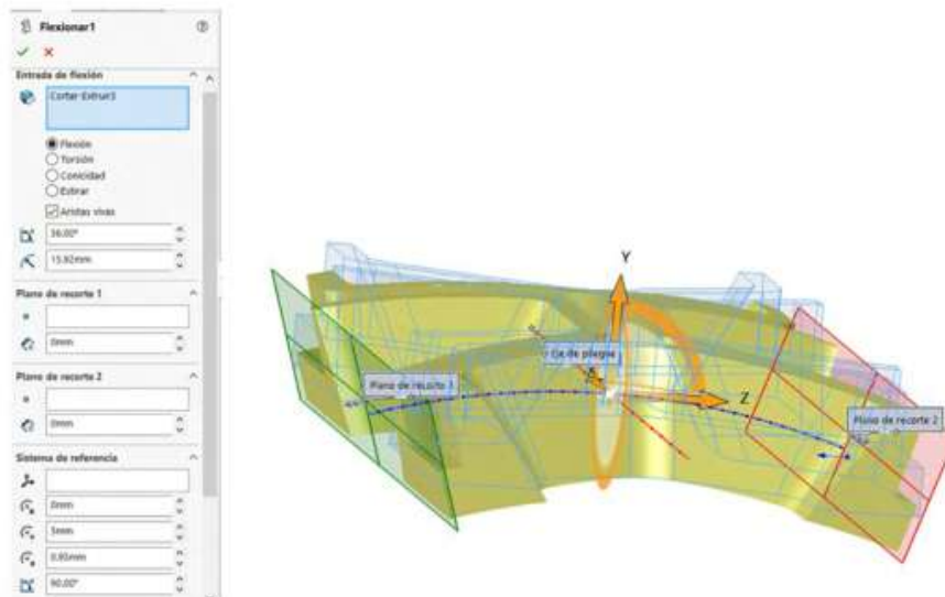
Figura 4.65. Realizar render con aplicación de materiales
