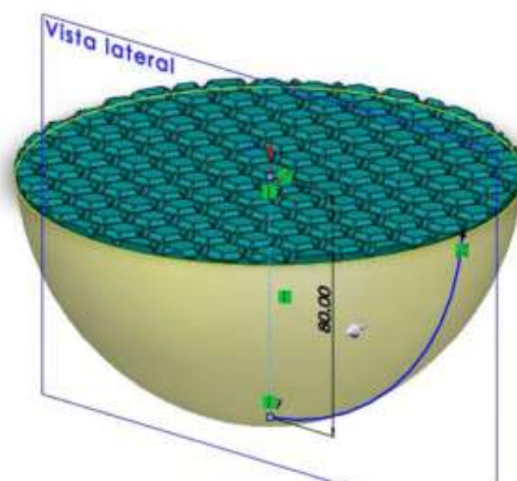
Figura 7.10. Mediante línea constructiva realizar revolución
