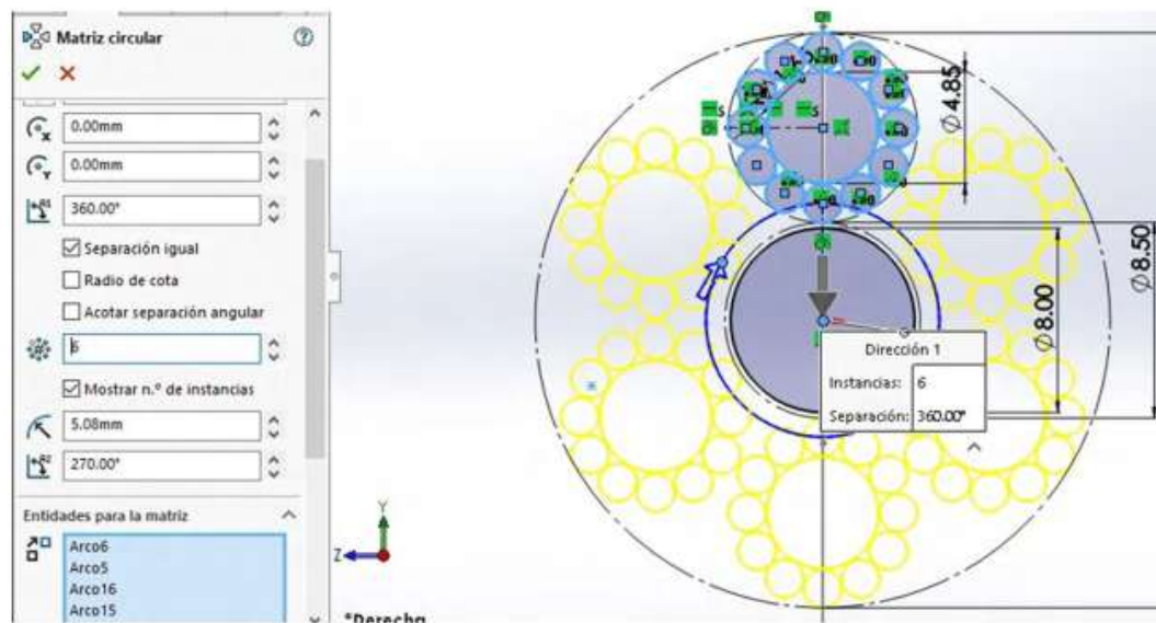
Figura 2.6. Matriz del patrón de la matriz inicial
