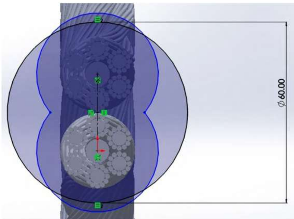
Figura 2.9. Croquis y dimensiones
