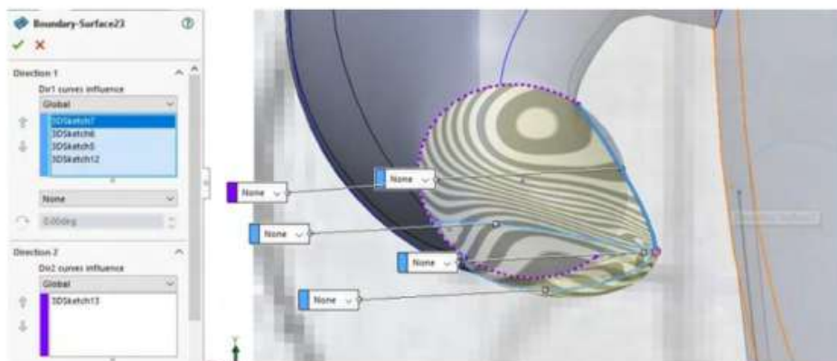
Figura 11.88. Realizar operación de rellenar por superficie
