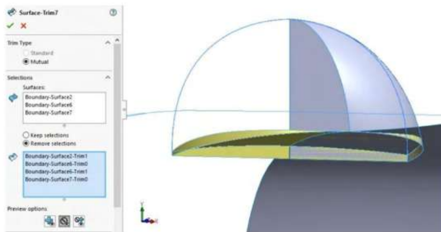
Figura 11.45. Recortar por superficie
