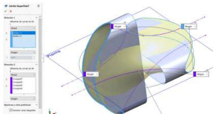
Figura 11.9. Mediante técnica de límite por superficie
