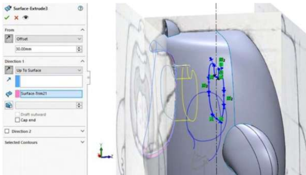
Figura 11.100. Seguir recortando superficie y coser
