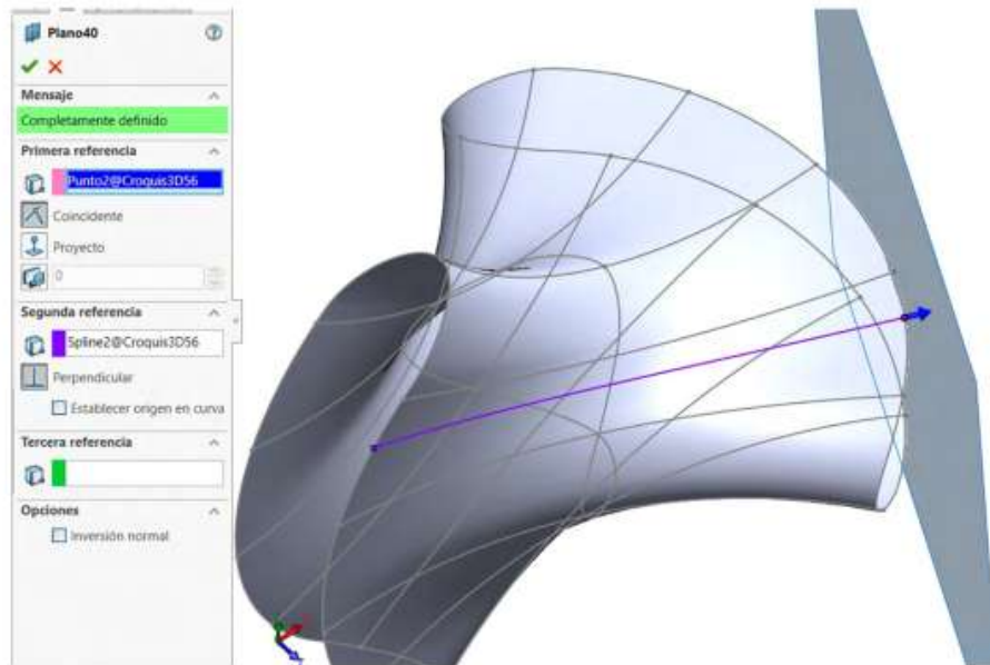
Figura 11.14. Realizar operación para un tercer plano
