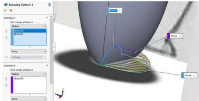
Figura 11.73. Generar operación de superficie por limitante
