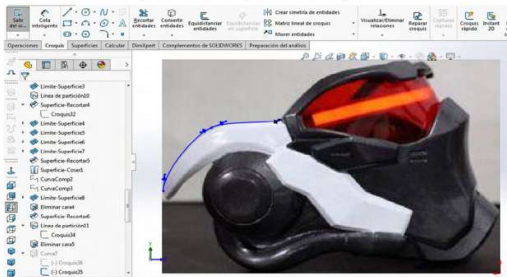
Figura 1.90. Mediante plano vista lateral y curva
