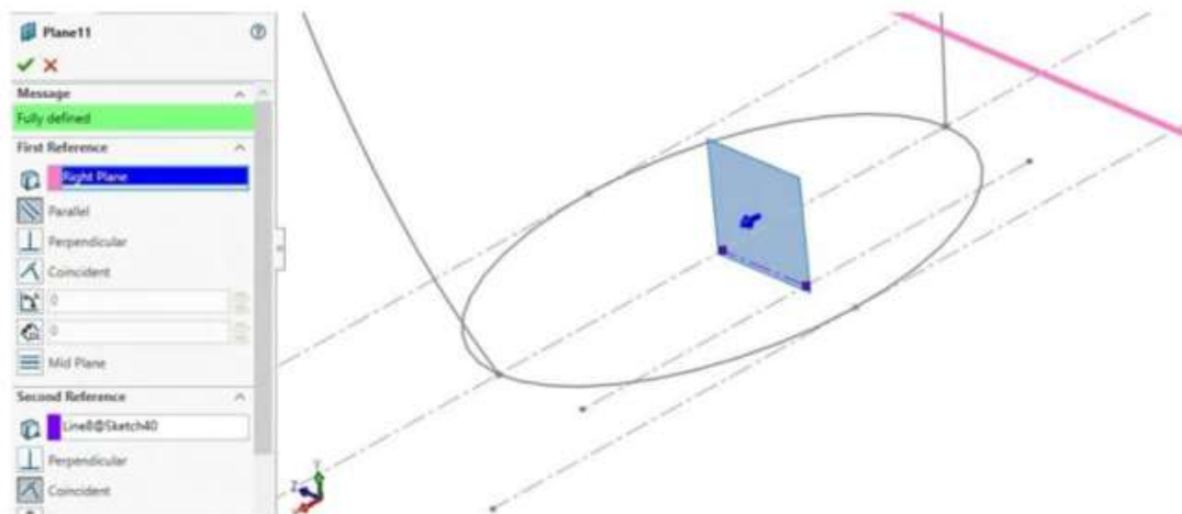
Figura 11.61. Genera plano mediante una vista lateral y línea auxiliar
