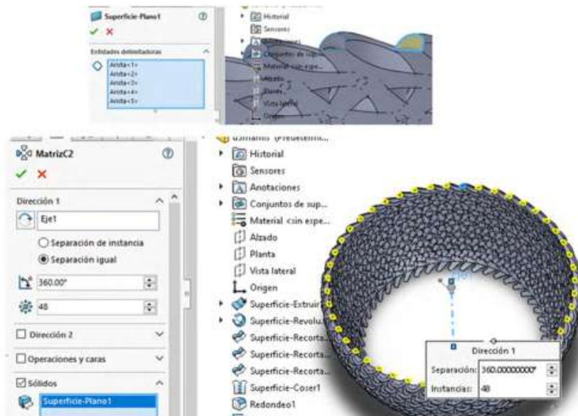
Figura 6.23. Completar matriz circular
