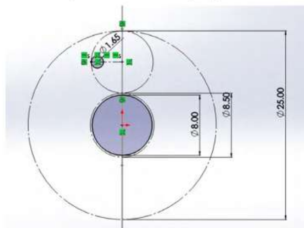
Figura 2.3. Dimensiones y trayectoria
