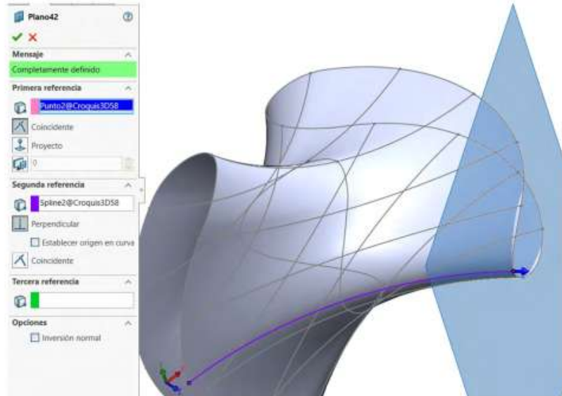
Figura 11.16. Repetir operación para un quinto plano
