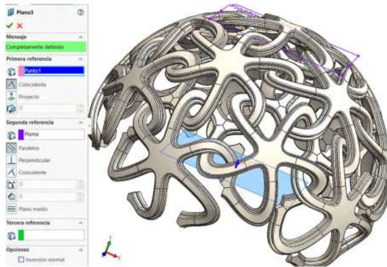
Figura 10.48. Generar plano nuevo
