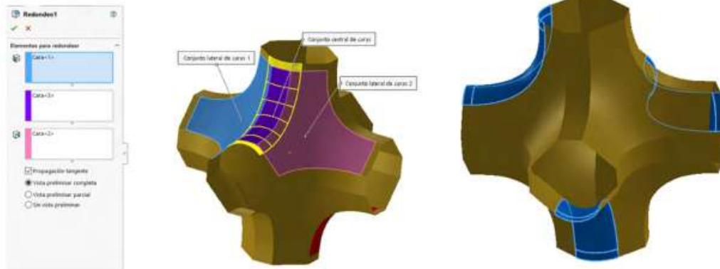
Figura 9.13. Aplicar redondeo por caras
