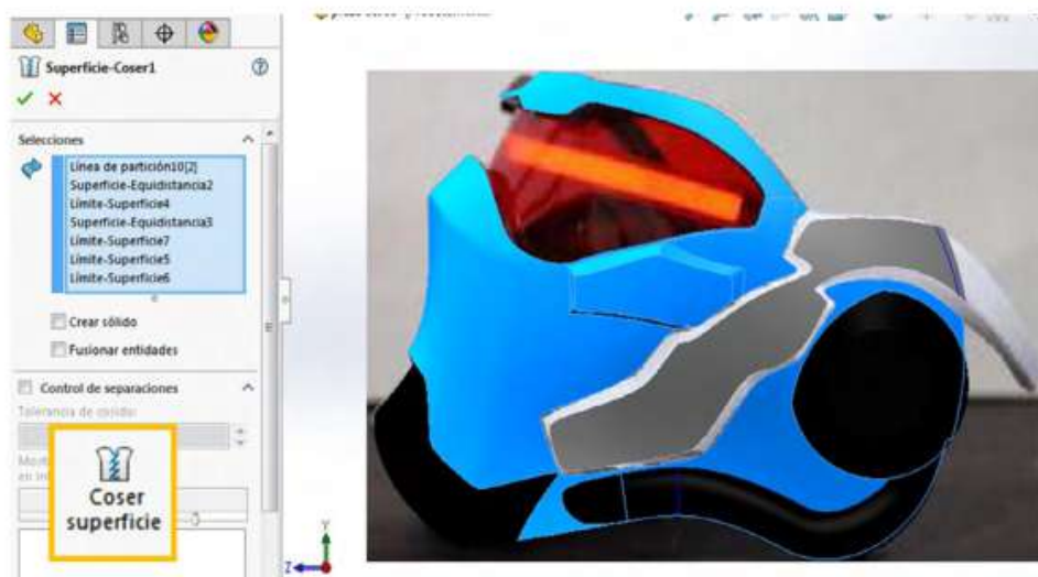
Figura 1.80. Mediante la opción de coser superficie
