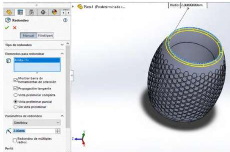
Figura 3.25. Realizar redondeos parte superior
