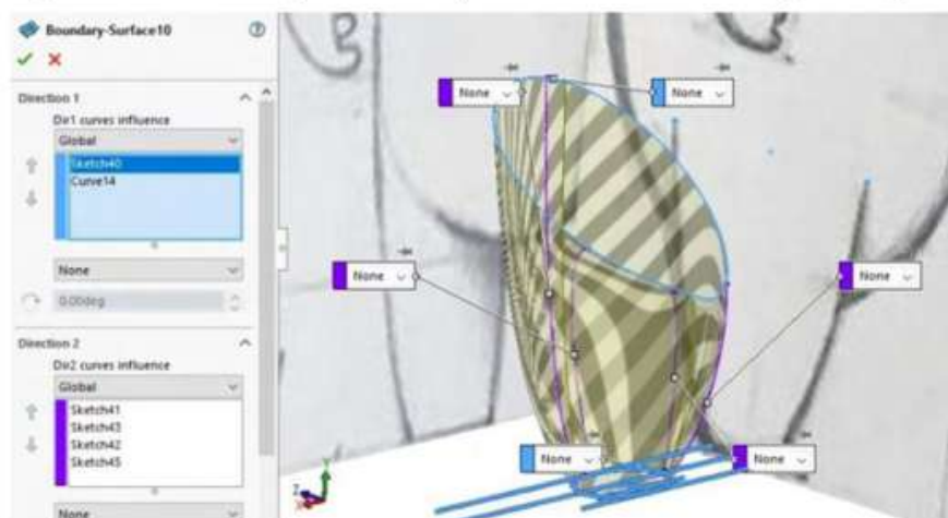
Figura 11.68. Realizar operación de superficie mediante limitante y curvas guías
