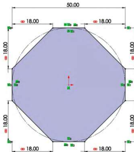
Figura 9.2. Realizar croquis y dimensiones
