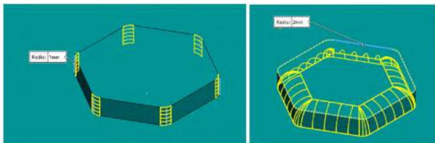
Figura 7.4. Realizar redondeos en aristas
