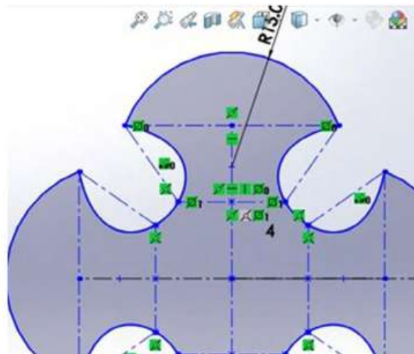
Figura 3.35. Realizar matriz circular para croquis
