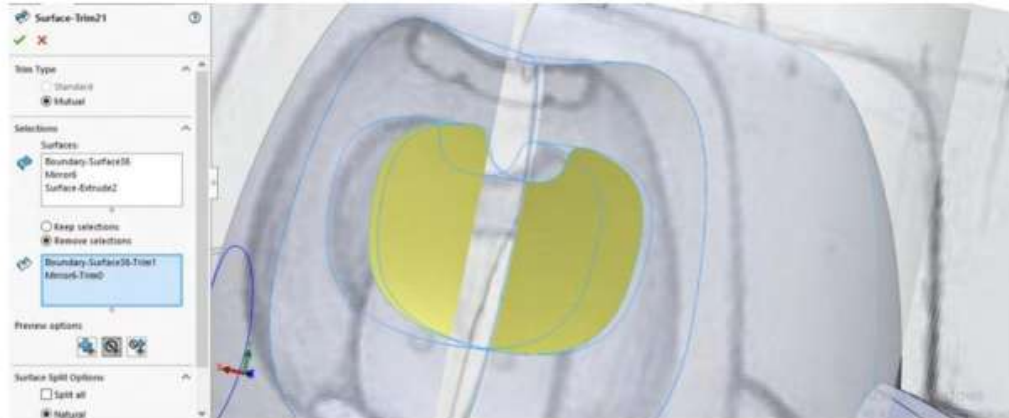
Figura 11.99. Recortar partes externas
