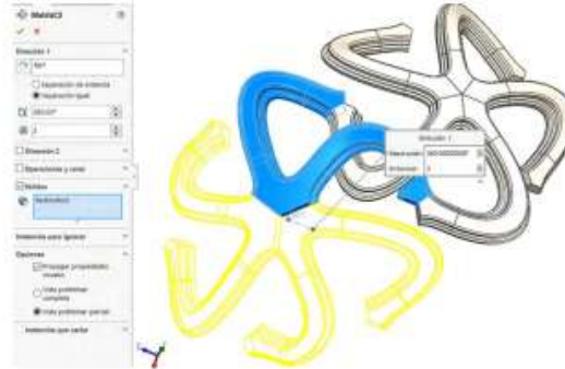
Figura 10.41. Aplicar una segunda matriz circular
