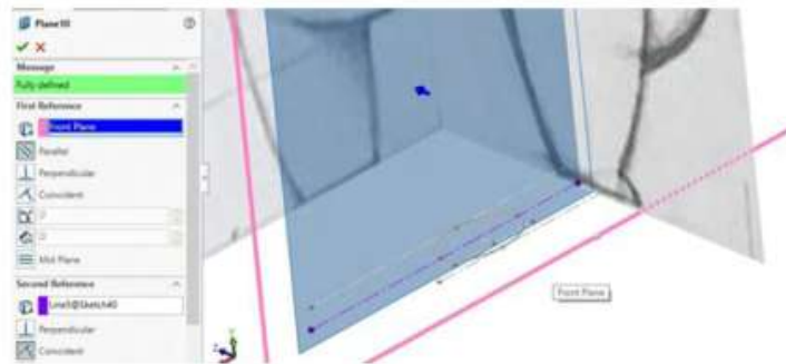
Figura 11.62. Visualizar posición del plano
