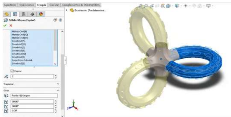
Figura 9.22. Mediante operación mover/copiar y opción en ángulo
