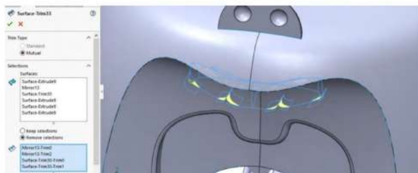
Figura 11.124. Retirar caras externas por recortar superficie
