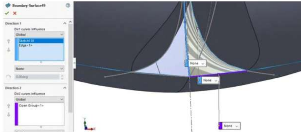
Figura 11.136. Realizar operación de recubrir por limitante
