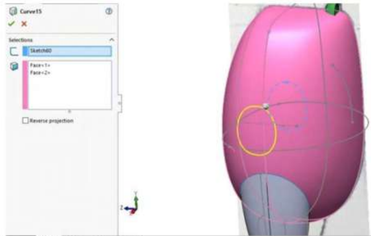
Figura 11.79. Proyectar curva a superficie
