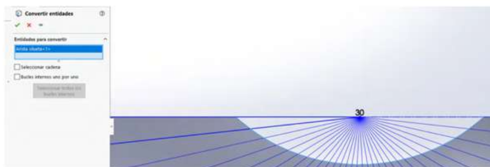
Figura 5.18. Equidistancia de entidades y convertir entidades
