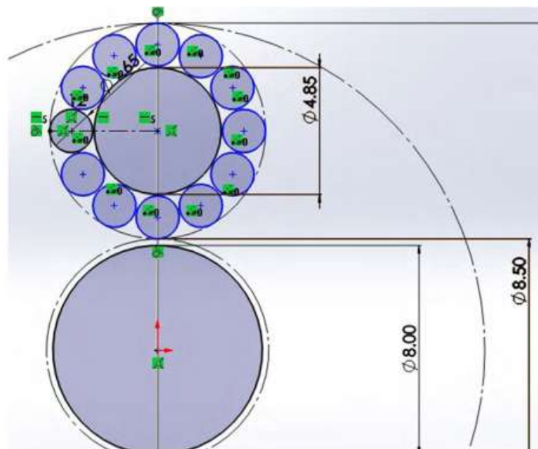
Figura 2.5. Dimensiones y matriz
