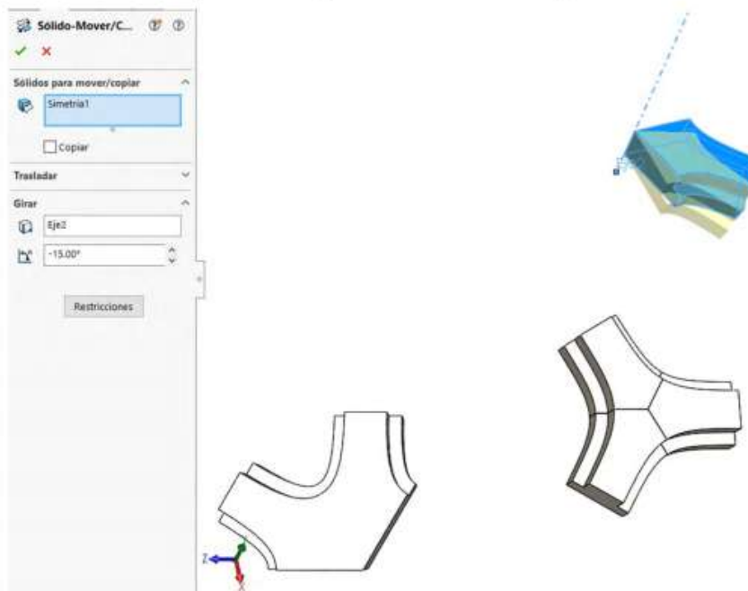
Figura 10.32. Aplicar movimiento en ángulo
