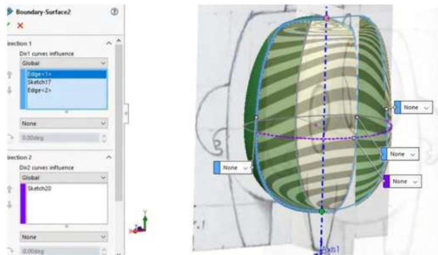
Figura 11.36. Crear superficie por límite con auxiliar de curvas
