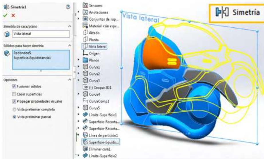
Figura 1.135. Mediante la opción de simetría
