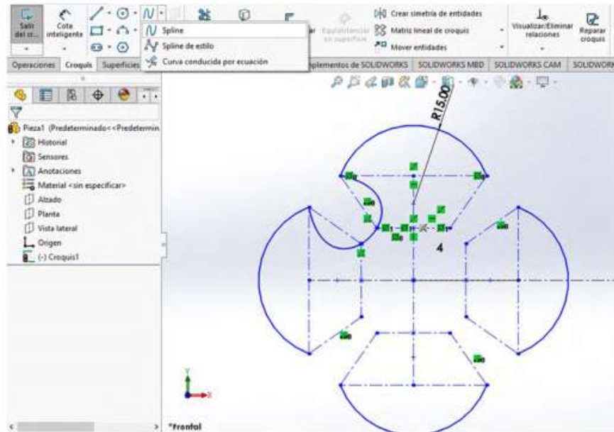
Figura 3.34. Realizar croquis mediante spline
