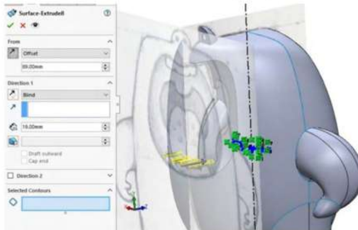
Figura 11.114. Realizar extruir por superficie
