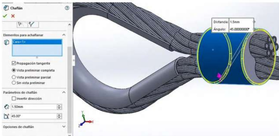
Figura 2.21. Operaciones de chaflán para quitar filo
