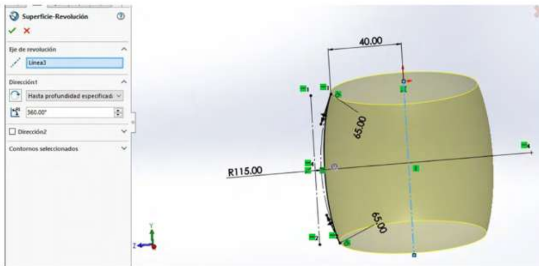
Figura 3.13. Dimensionar y aplicar revolución
