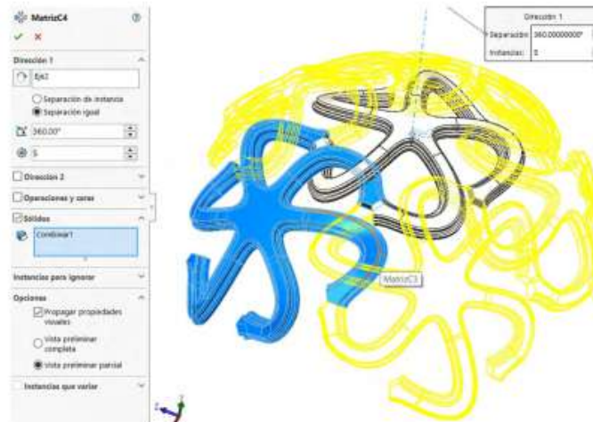
Figura 10.44. Aplicar matriz circular
