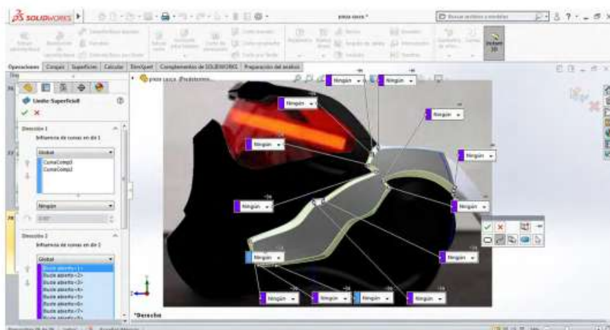
Figura 1.84. Mediante la opción de superficie limitante
