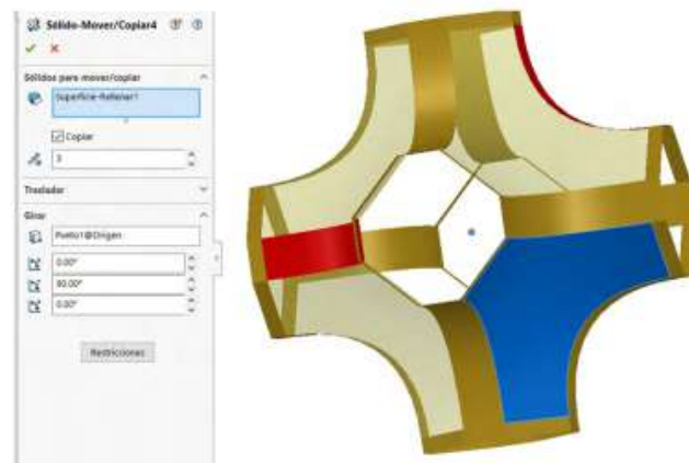
Figura 9.11. Aplicar operación de mover/copiar mediante opción ángulo
