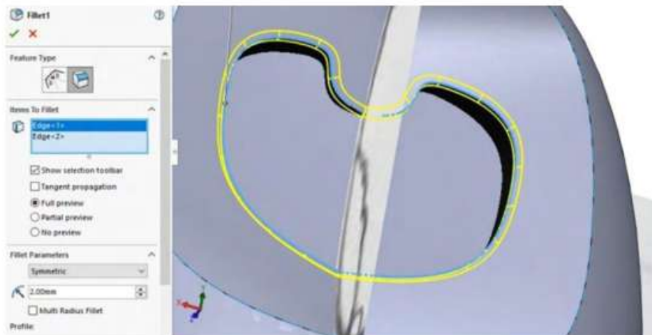
Figura 11.101. Aplicar redondeo en aristas
