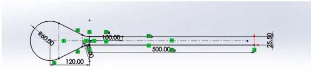
Figura 2.2. Croquis y dimensiones de ruta
