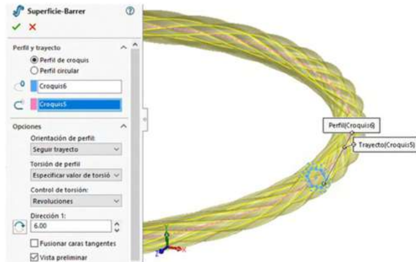
Figura 6.28. Realizar un barrido por superficies
