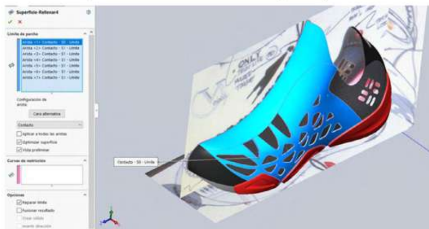
Figura 8.49. Realizar un relleno de cuerpo en superficie
