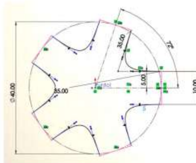
Figura 10.11. Mediante plano planta realizar croquis
