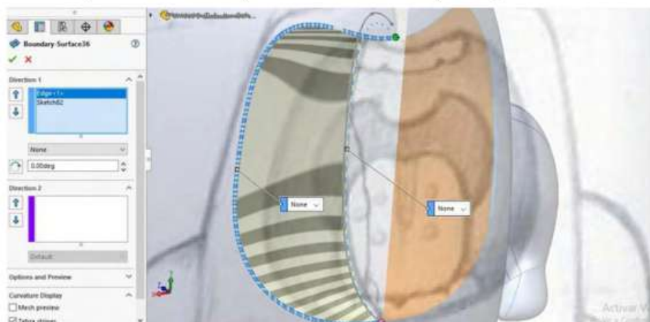
Figura 11.96. Realizar operación de recubrir en superficie por limitante
