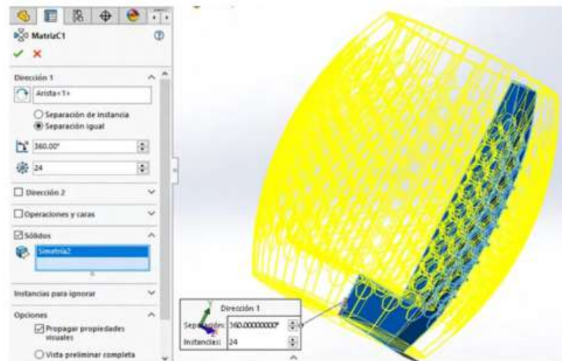
Figura 3.21. Realizar matriz circular
