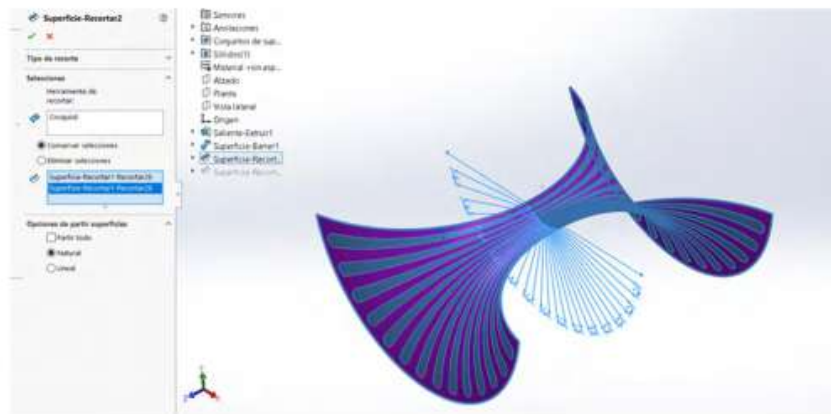
Figura 5.22. Recorte por superficie
