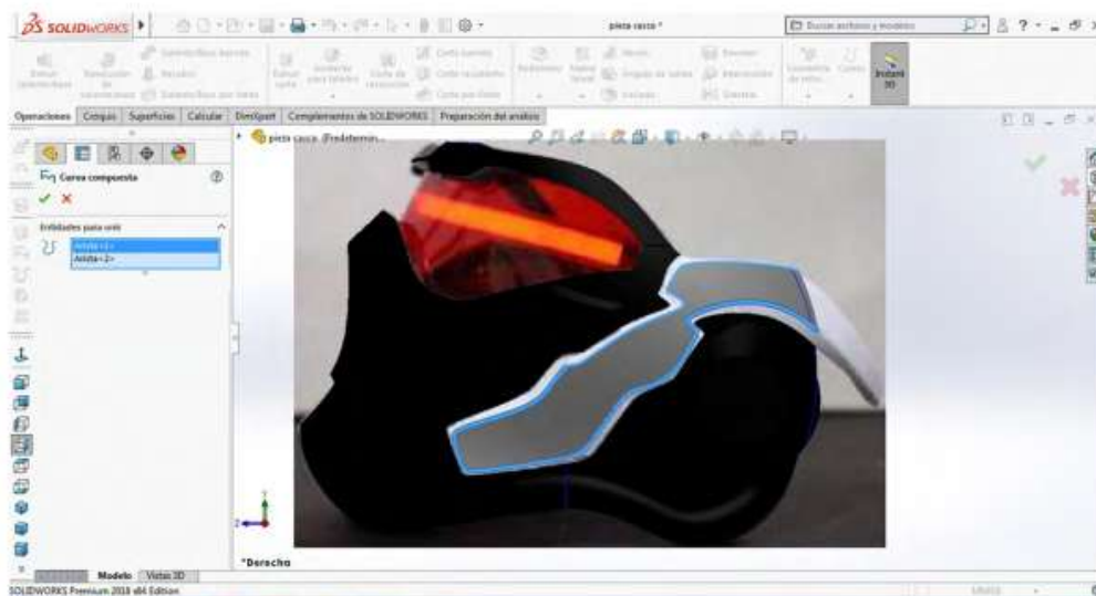
Figura 1.82. Mediante la opción de curva compuesta y selección de aristas
