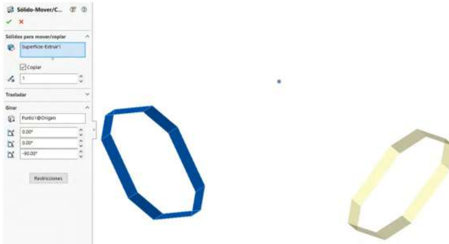
Figura 9.4. Operación mover/copiar mediante opción de ángulo
