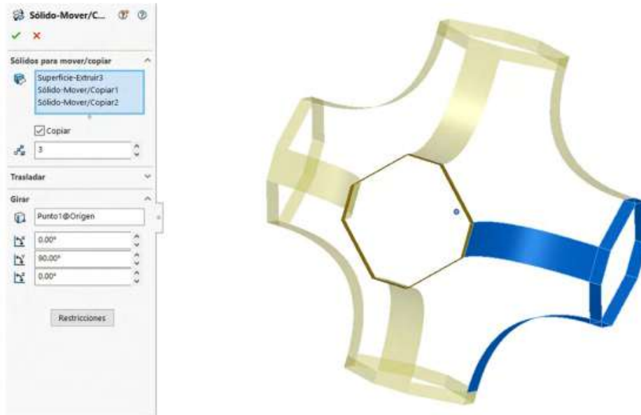
Figura 9.8. Repetir operación cambiando el eje
