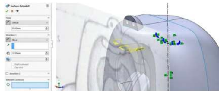
Figura 11.123. Aplicar operación extruir por superficie
