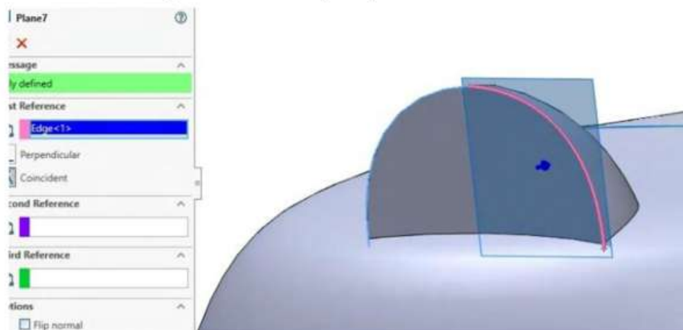
Figura 11.46. Generar plano por arista de referencia
