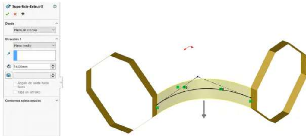
Figura 9.6. Realizar extruir por plano medio
