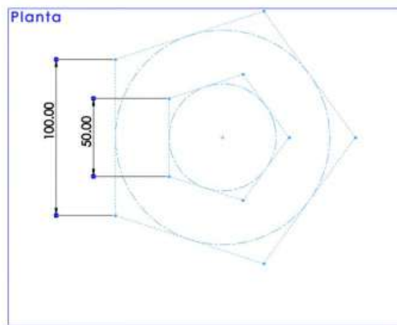
Figura 10.2. Croquizando con dimensiones
