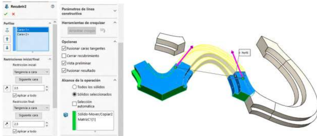
Figura 10.37. Recubrir cuerpos faltantes
