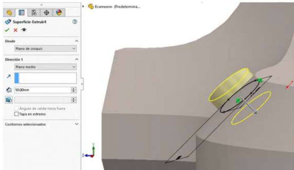
Figura 9.18. Realizar operación extruir por plano medio
