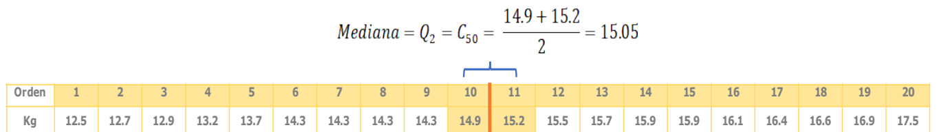
Figura 22. Cuartil 2 ( Q_2 )
