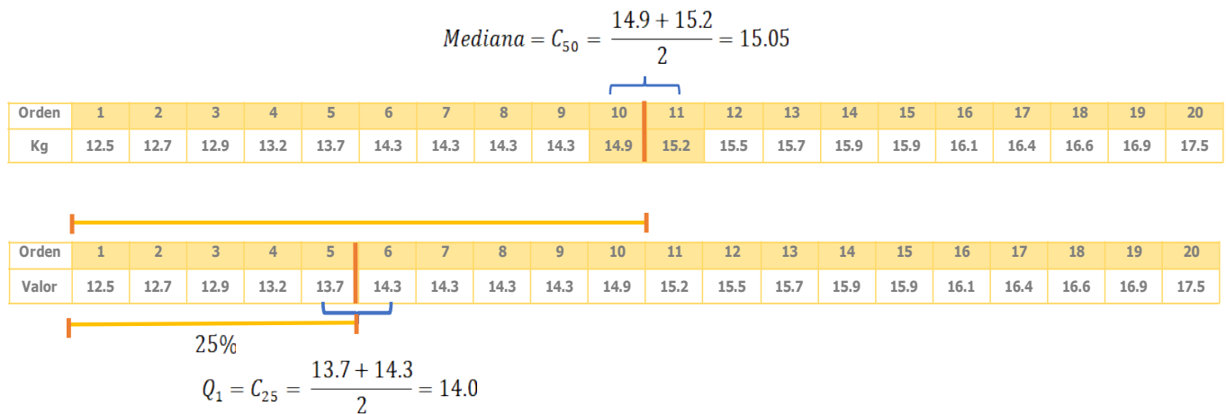
Figura 21. Cuartil 1 ( Q_1 )
