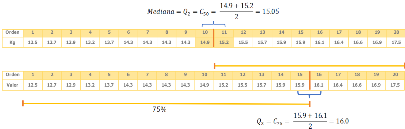
Figura 23. Cuartil 3 ( Q_3 )
