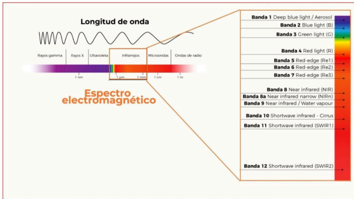
Figura 5.5. Representación del espectro electromagnético en el cual las imágenes de satélite capturan la información de la superficie, el sensor Sentinel-2, del programa Copernicus, tiene 13 bandas diferentes. Fuente: Modificado de https://www.edu-sat.com/ .
