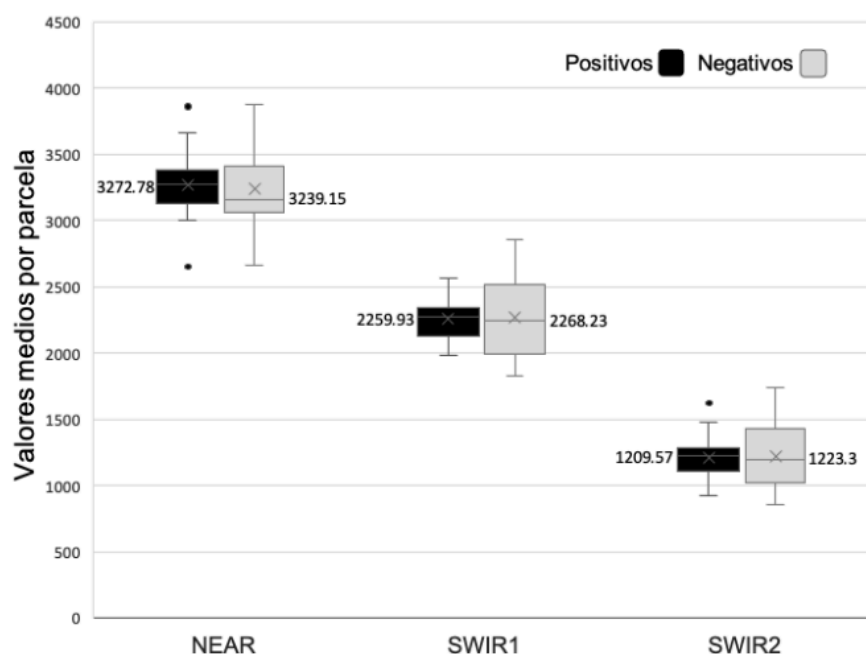
Gráfica 5.2. Resumen de las estadísticas de las bandas cinco, seis y siete del satélite Landsat 8 calculados para las parcelas con categoría Positiva (con HLB) y Negativas (sanas).
