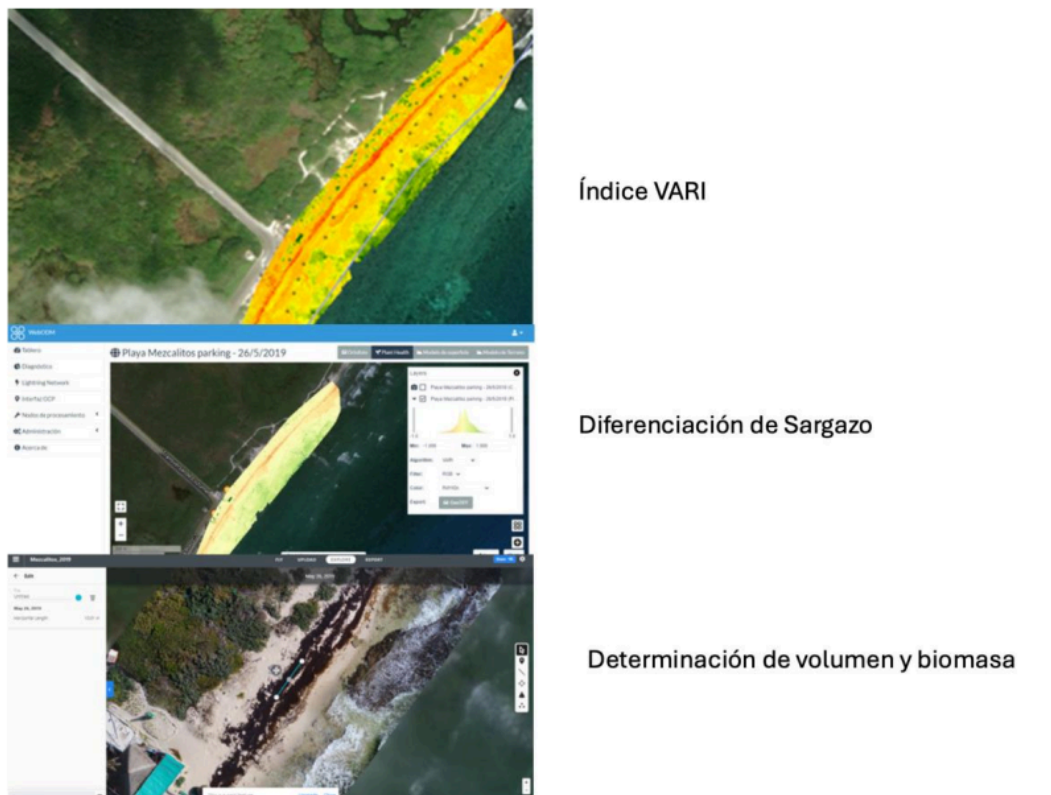
Figura 6.6. Reconocimiento del índice VARI, Diferenciación de Sargazo y Determinación de volumen y biomasa en playa Mezcalitos en 2019.
