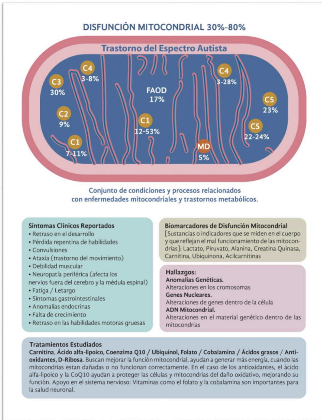
Figura 14. Características importantes de la disfunción mitocondrial asociada con el trastorno del espectro autista (TEA). Fuente: basado en Richard E. Frye (2020). Elaboración propia. (Gráfica original en Anexo 4).
