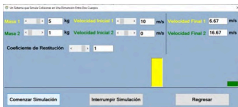
Figura 3.7. Ventana que muestra la colisión cuando una masa es cinco veces mayor que la otra
