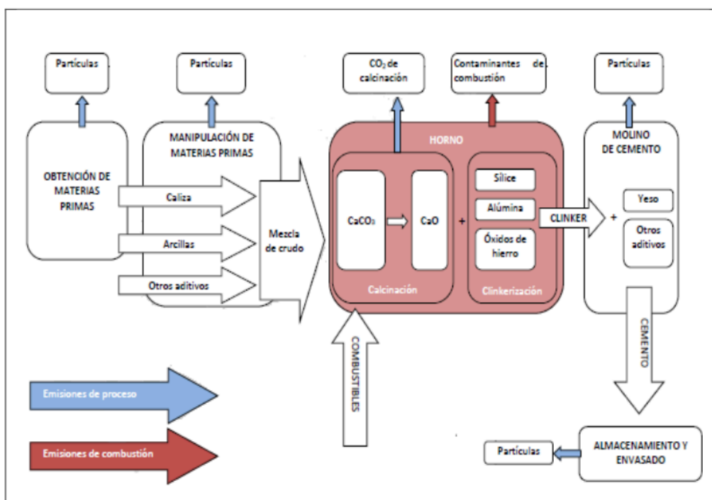
Figura 4.-La liberación de CO 2 a lo largo del ciclo de producción de cemento
